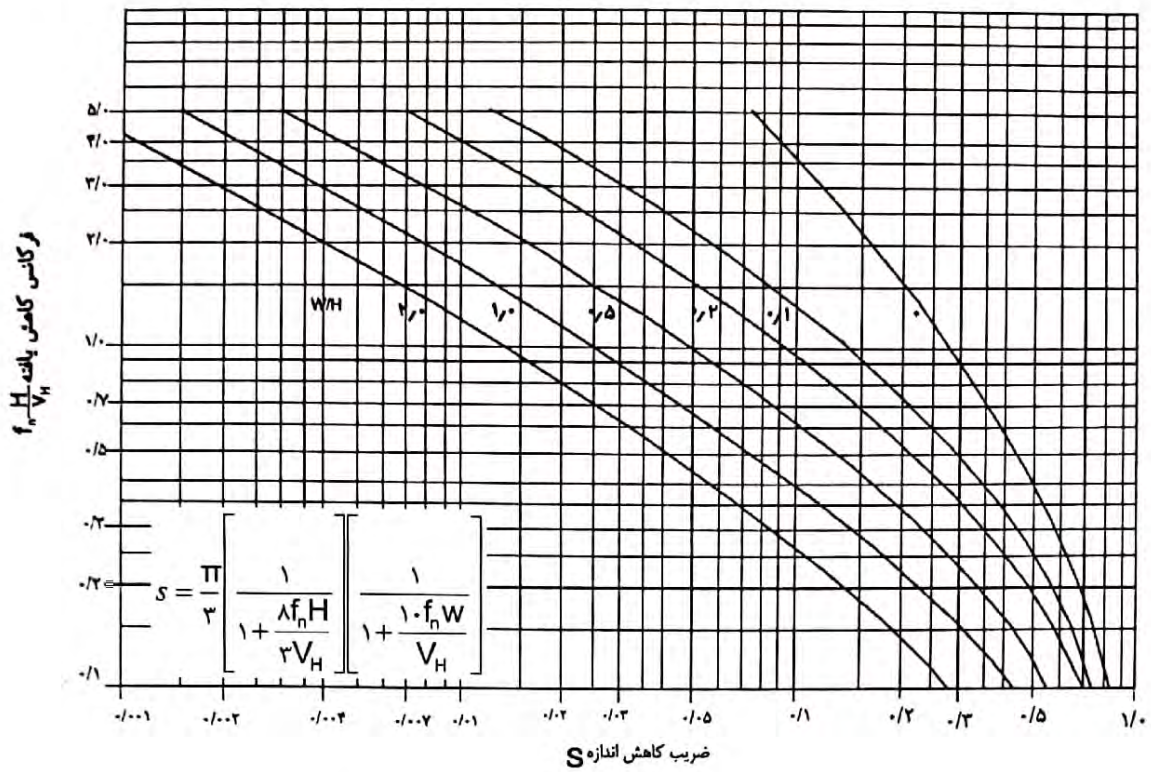
شکل پ-۴-۶-۲ ضریب کاهش اندازه (S)
