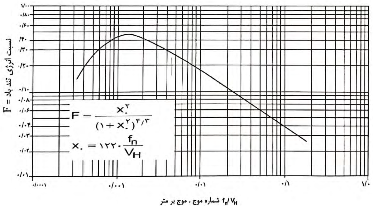
شکل پ-۴-۶-۳ نسبت انرژی تندباد (F)
