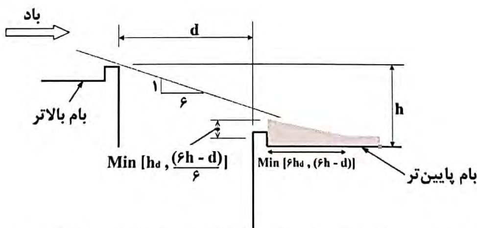
شکل ۶-۹-۷-۲ بار انباشتگی برف پشت به باد روی بام پایین تر ساختمان مجاور
