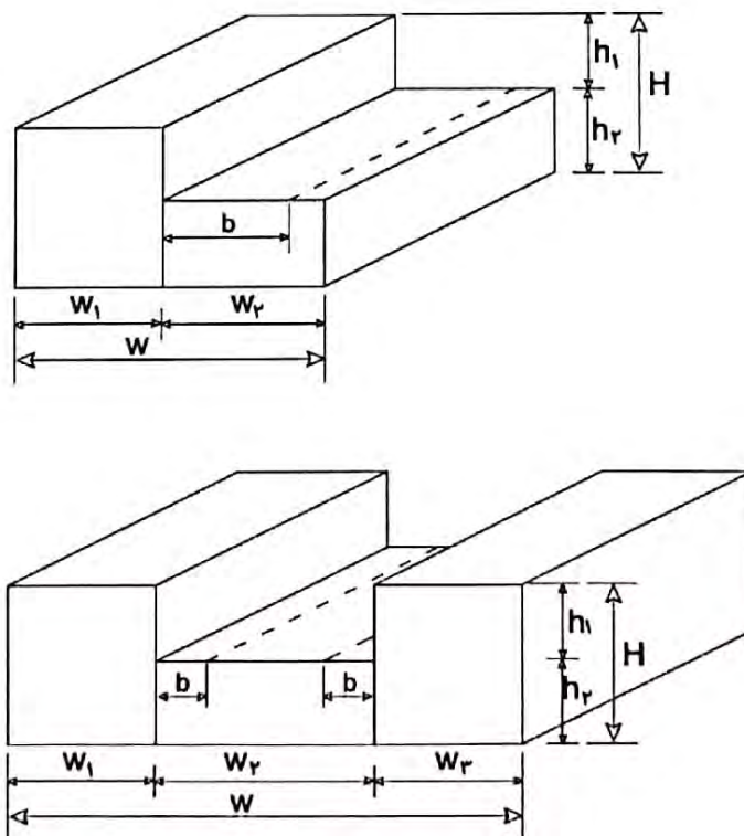
شکل ۶-۱۰-۱۱ نسبت ابعادی ساختمان‌های با بام پله‌ای تخت
